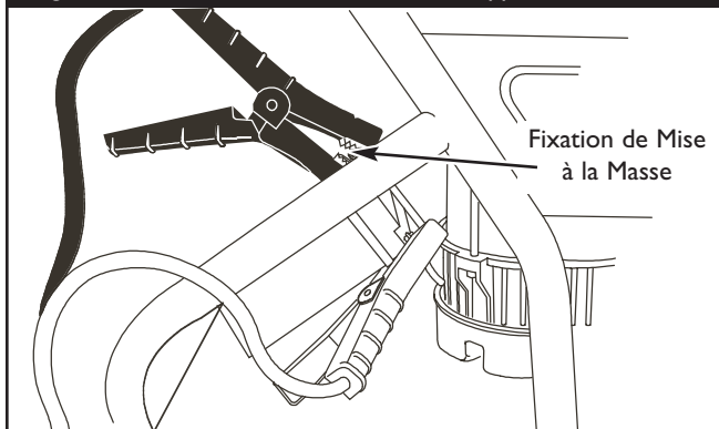
Figure 23 — Branchement des Câbles d'Appoint
